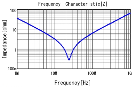
■ DE2E3SA472MA3BX02F |Z| DCOV, 20degC
