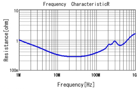
■ DE2E3SA472MA3BX02F R DCOV, 20degC
