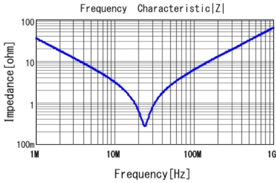
■ DE2E3SA472MA2BT01F |Z| DCOV, 20degC
