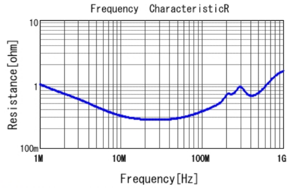
■ DE2E3SA472MA2BT01F R DCOV, 20degC
