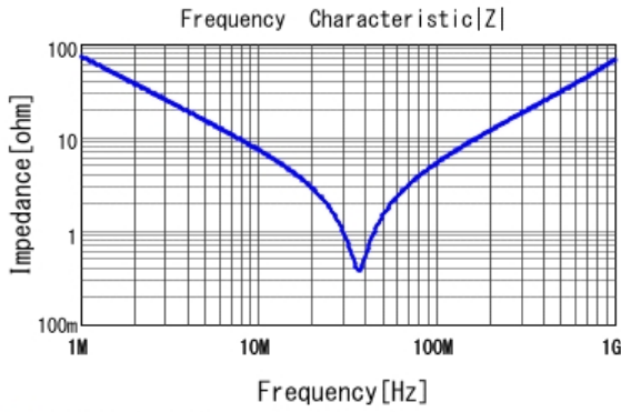
■ DE2E3SA222MJ3BT02F |Z| DCOV, 20degC
