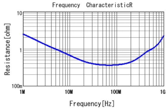
■ DE2E3SA222MJ3BT02F R DCOV, 20degC
