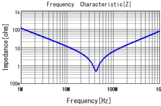
■ DE2E3SA152MA2BT01F |Z| DCOV, 20degC
