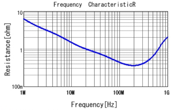
■ DE2E3SA102MJ3BT02F R DCOV, 20degC
