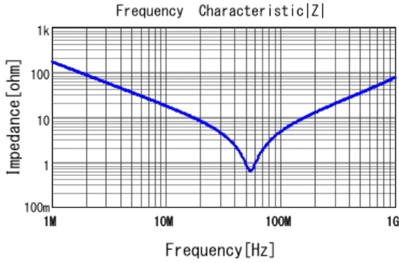
■ DE2E3SA102MJ3BT02F |Z| DCOV, 20degC
