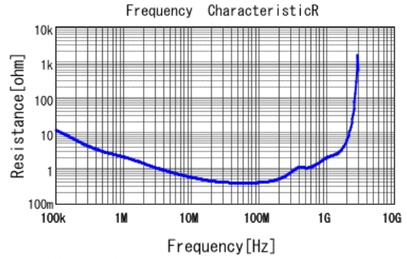
■ DE2E3KY332MN3AM02F R DCOV, 20degC
