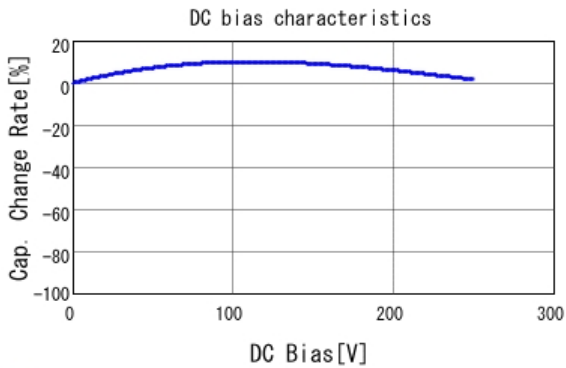
■ DE2E3KY332MN3AM02F C-DC bias capchange, 20.0degC, AC1
