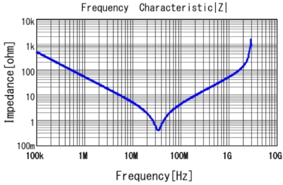
■ DE2E3KY332MN3AM02F |Z| DCOV, 20degC
