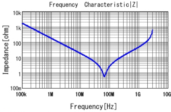
■ DE2E3KY102MN3AU02F |Z| DCOV, 20degC
