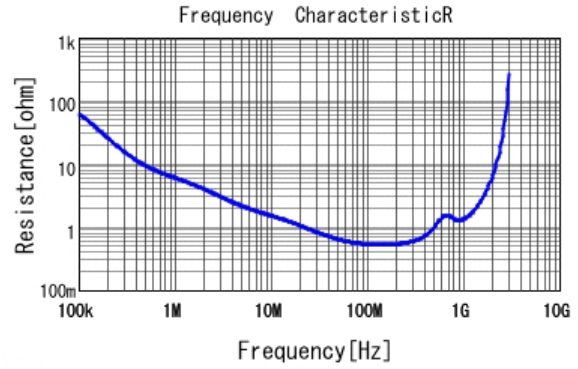
■ DE2E3KY102MN3AU02F R DCOV, 20degC
