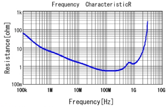
■ DE2E3KY102MB3BM02F R DCOV, 20degC
