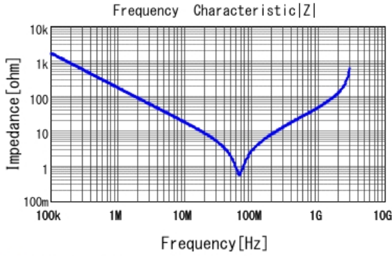
■ DE2E3KY102MB3BM02F |Z| DCOV, 20degC
