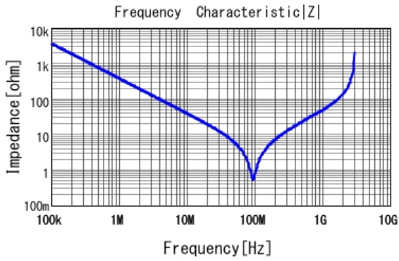
■ DE2B3KY471KA3BU02F |Z| DCOV, 20degC
