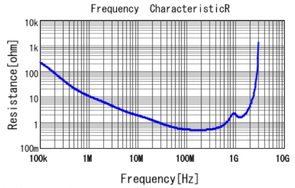
■ DE2B3KY471KA3BU02F R DCOV, 20degC
