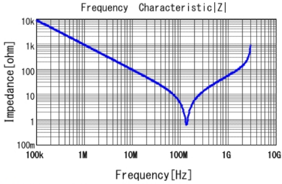
■ DE2B3KY221KA3BU02F |Z| DCOV, 20degC
