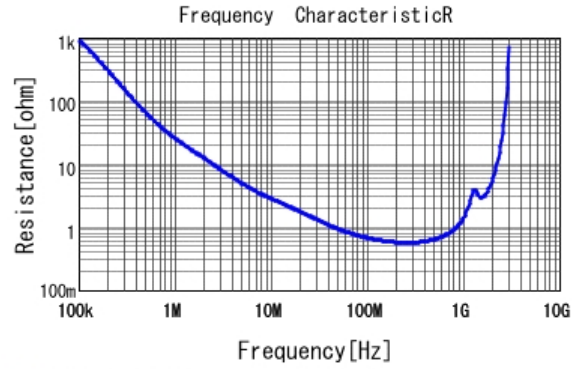
■ DE2B3KY221KA3BU02F R DCOV, 20degC
