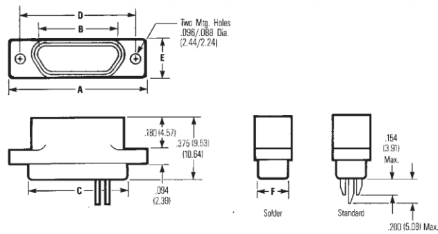
Socket
