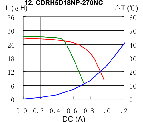
12. CDRH5D18NP-270NC
