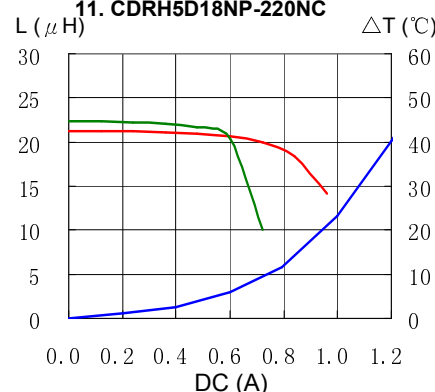
11. CDRH5D18NP-220NC
