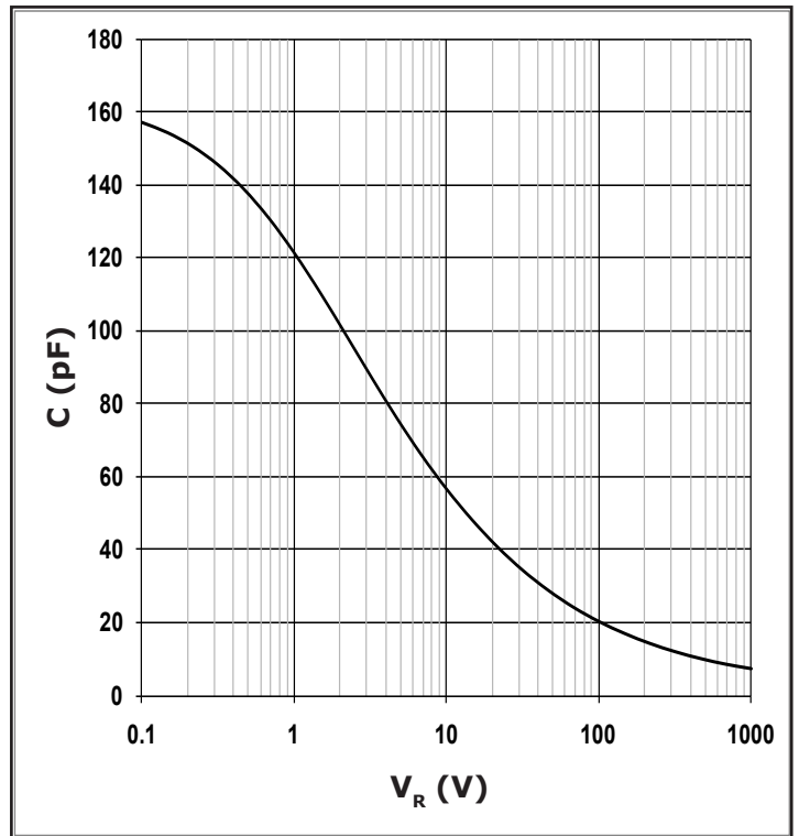
图 6. 电容与反向电压
