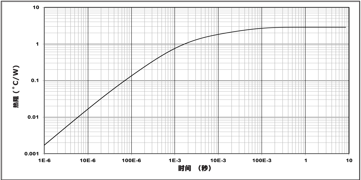
图 7.瞬态热阻抗
