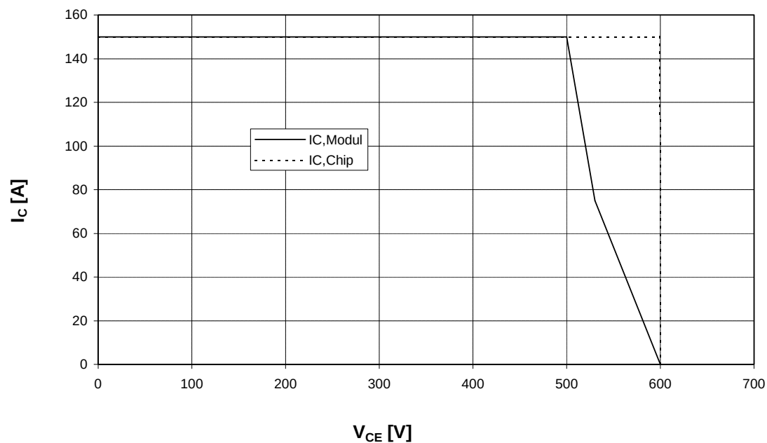
Sicherer Arbeitsbereich Wechselr. (RBSOA)
