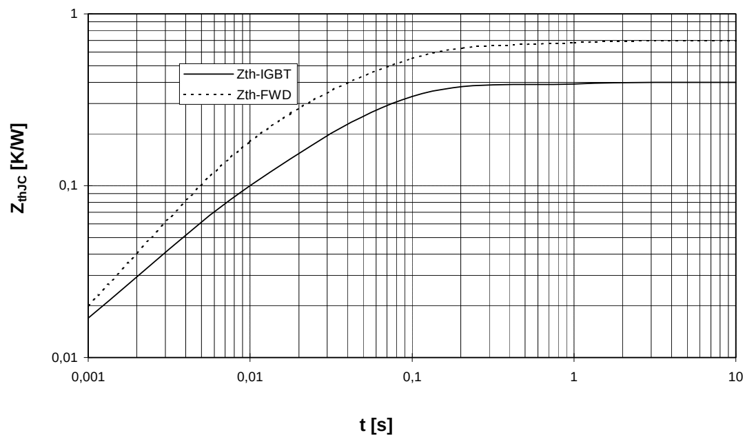
Transienter Wärmewiderstand Wechselr. Transient thermal impedance Inverter
