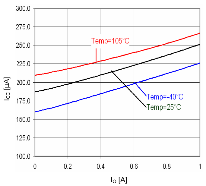
Fig.32 Io-Icc
