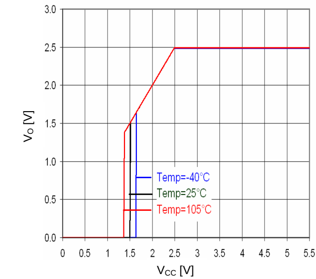
Fig.27 V_{cc} - V_o ( I_o=0\text{mA} )
