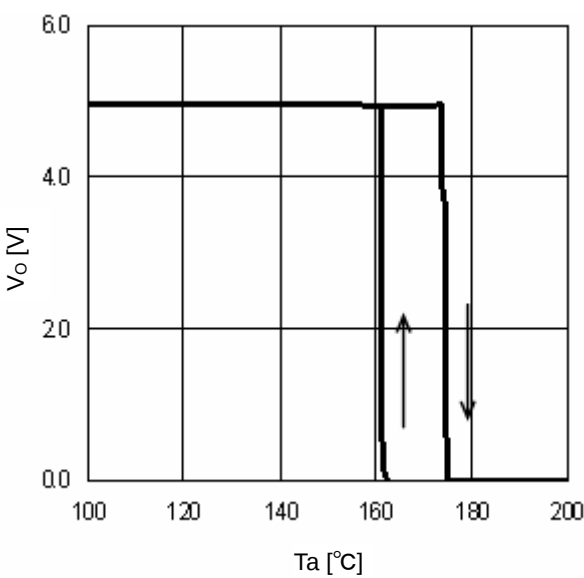
Fig.28 TSD ( I_o=0\text{mA} )
