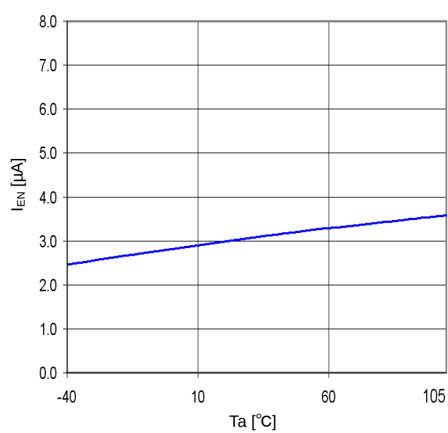
Fig.24 T_a - I_{EN}
