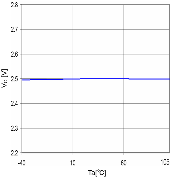
Fig.21 T_a-V_o (I_o=0mA)
