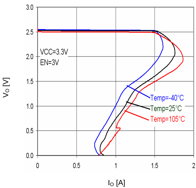
Fig.29 I_o - V_o
