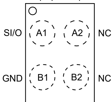
4-Ball WLCSP (Top View)
