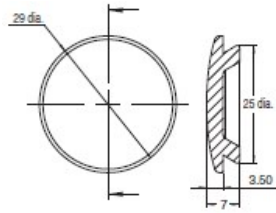
A22NZ-A-401
