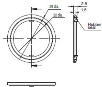
A22NZ-A-403
