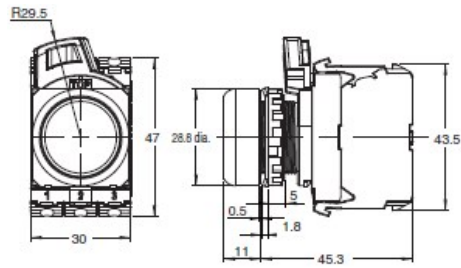
A22NN-RN[]-N[]A-G[]-NN
