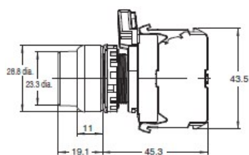
A22N[]-RP[]-[]A-G[]-[]
