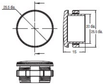
A22NZ-A-402
