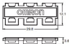
A22NZ-A-C01
