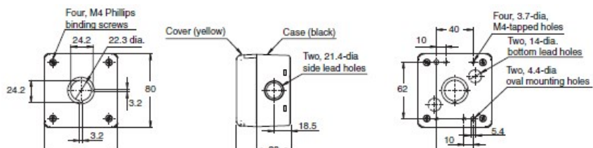
A22NZ-A-B01Y
