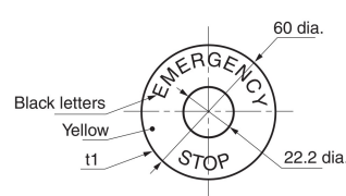
A22Z-3466-1 (60 dia.)
