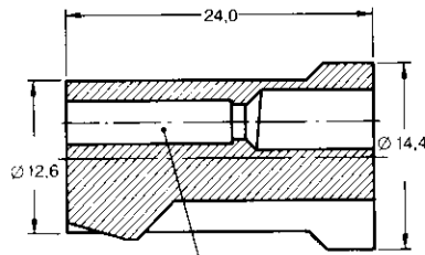
Kammer für CI 2 Kontakt Cavity for CI 2 Contact
