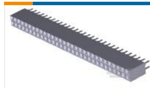
TE Part #8-147424-0 60 MODII VRT DR CE .100 X .100
