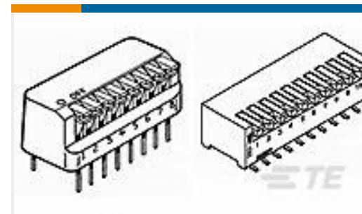
TE Part #435802-8 RIGHT ANGLE DIP SW 10 POS AU
