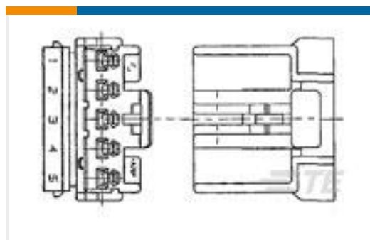
TE Part #347477-1 MULTILOCK RECEPTACLE HSG.5 WAY
