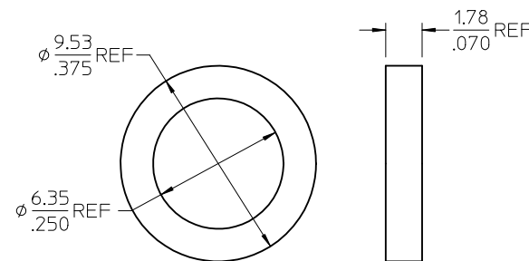
GASKET
