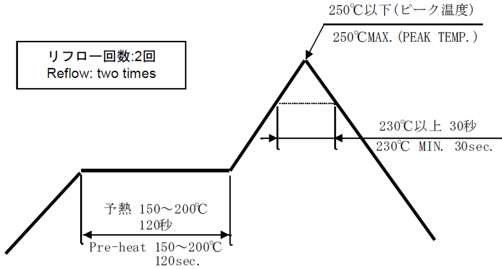
温度条件グラフ TEMPERATURE CONDITION GRAPH (はんだ接合部の基板表面にて測定)
