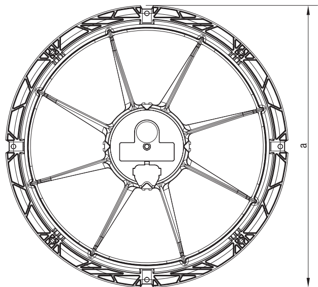
Type A: Round fan housing
