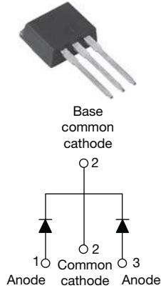
VS-42CTQ030-1PbF
