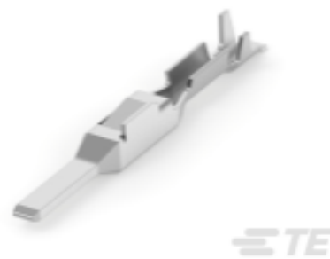
TE Part #2109005-3 060 TAB(M) CONT
