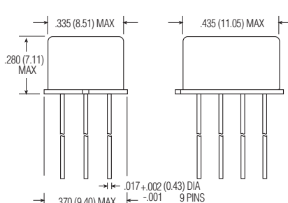
MGAT Enclosure
