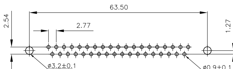
P.C.B. LAYOUT
