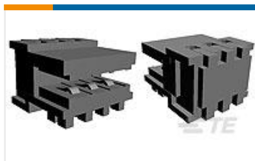
TE Part #3-829868-3 16X 3P FEDERLEI 2,5
