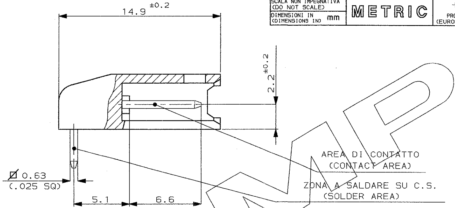
SEZ. PARZIALE (PARTIAL SEC.) A-A
