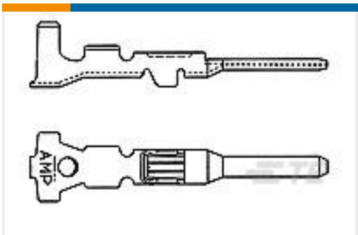
TE Part #282109-1 MINI MIC TAB CONTACT
