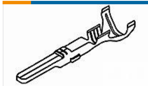
TE Part #171631-1 E-J MK-2 070 TAB CONT
