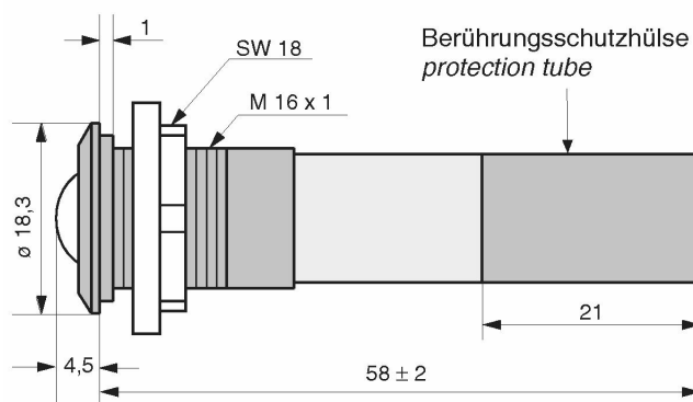
Flachdichtung / gasket
