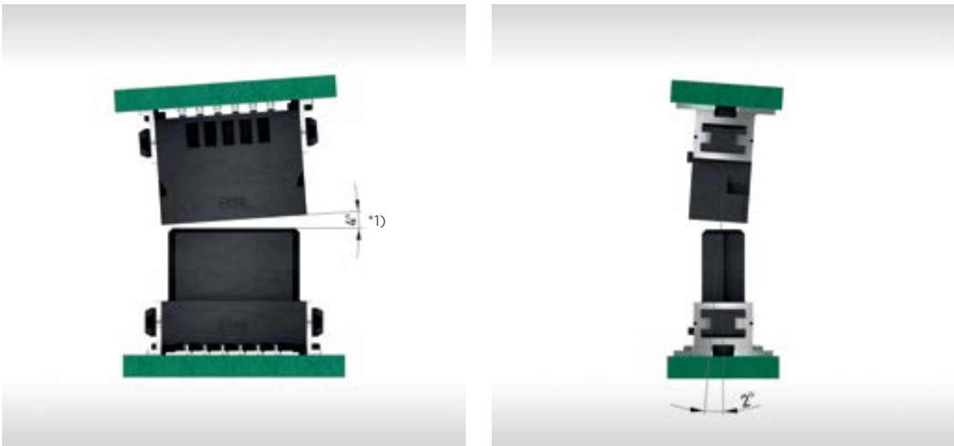
Zulässiger Winkelversatz für eine sichere Selbstzentrierung
