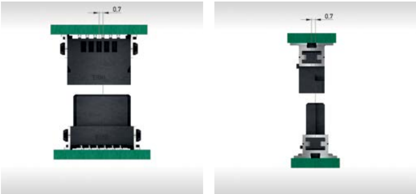
Zulässiger Mittenversatz für eine sichere Selbstzentrierung
