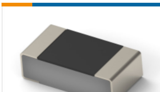
TE Part #5-1879808-7 RP 1J 0.1W 453K 0.1% 15PPM 1K RL
