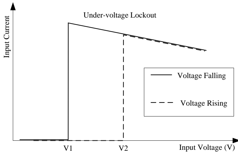
Figure 30. Input under-voltage lockout V1 = 44 V V2 = 47 V
